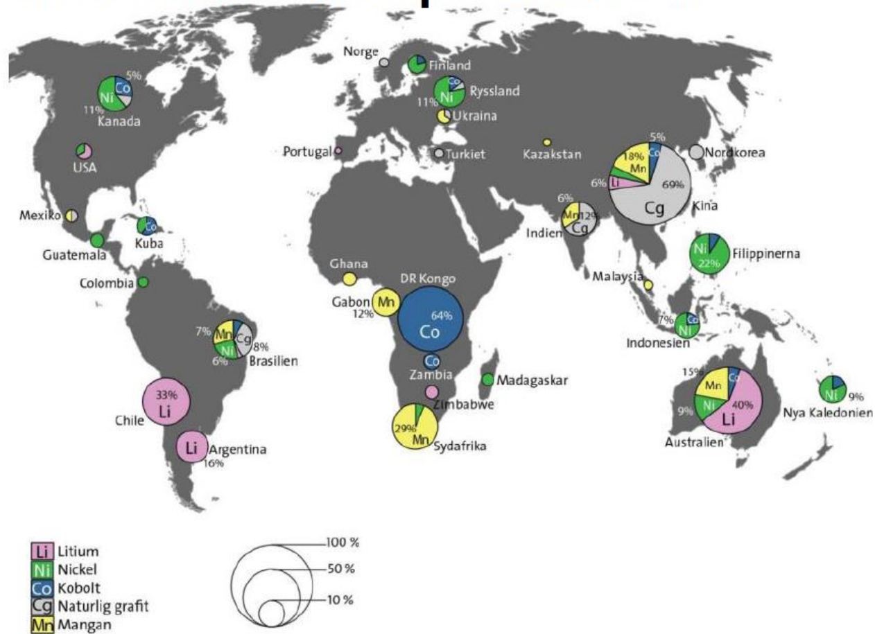
Figur 2. Världspåproduktion av batterimetaller (Layout: Lars Norlin SGU, källor: EU-kommissionen 2017b, USGS 2017, BGS 2016).
